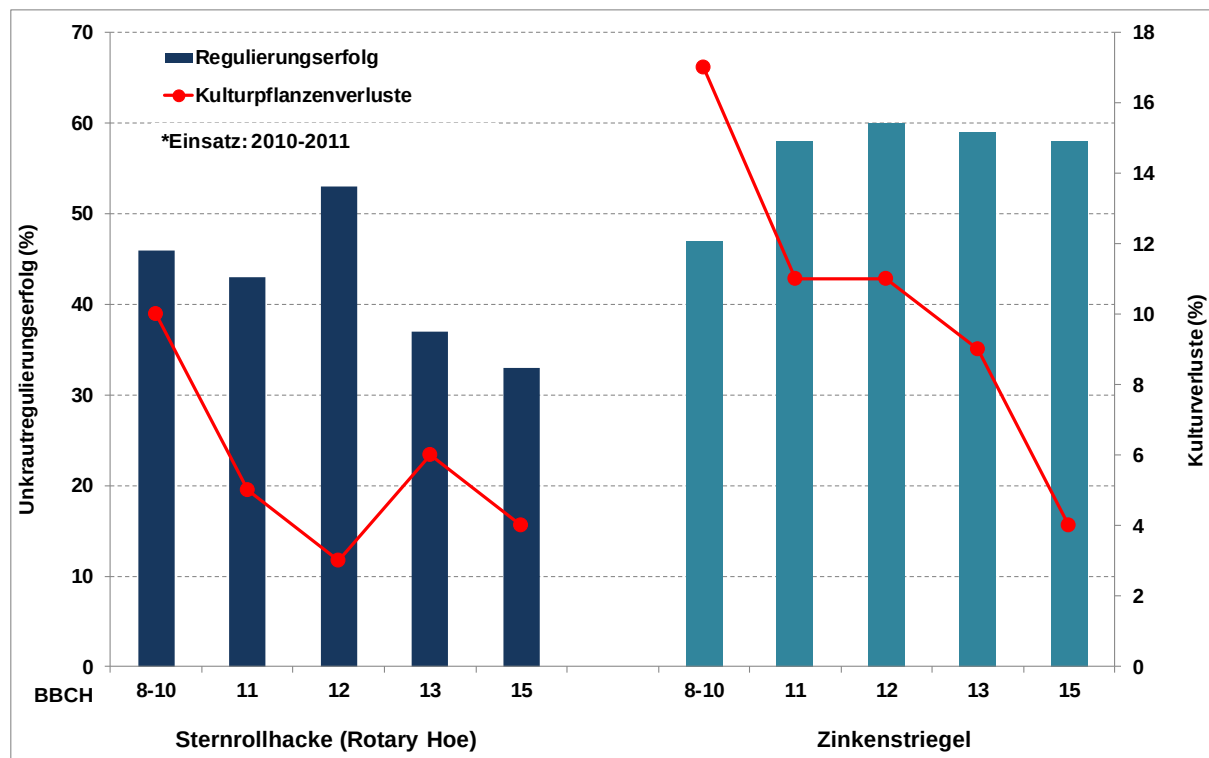
Abbildung 1: Regulierungserfolg und Kulturpflanzenverluste von Sternrollhacke und Zinkenstriegel – Mittelwerte 2009 bis 2011
