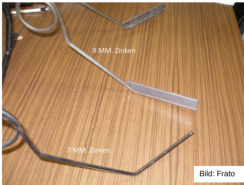
Abbildung: 28: Torsionshacke mit Häufelblechen
