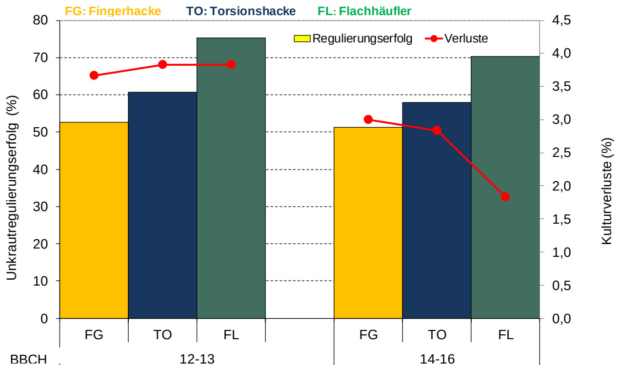
Abbildung 3: Regulierungserfolg und Kulturpflanzenverluste der reihenabhängigen Werkzeuge – Mittelwerte 2009 bis 2011
